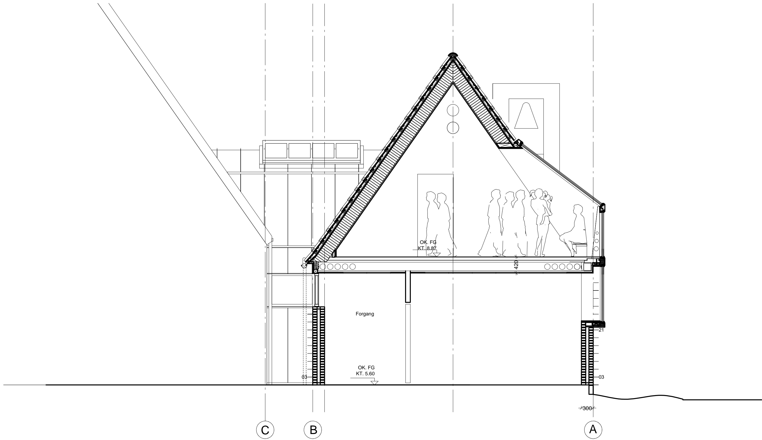
PRINCIP SNIT A-A
